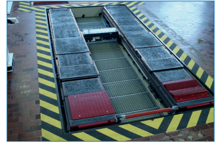
R-AS im Rechteckfundament mit (optionaler) Gitterberostung (Ausstattung für Fahrzeugprüfung).
