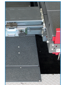
R-AS im Rechteckfundament mit (optionaler) Gitterberostung (Ausstattung für Fahrzeugprüfung).
